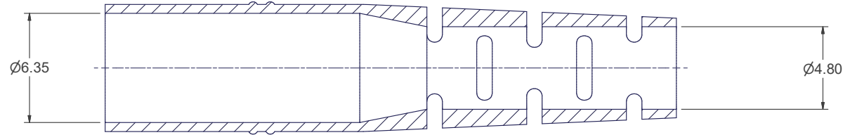
SECTION A-A
